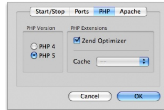
Nastavenie PHP
