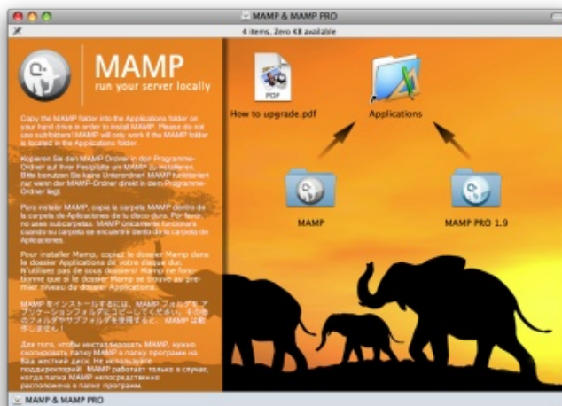
Inštalácia MAMPu
