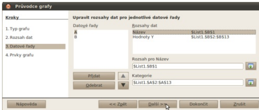
Datové řady
