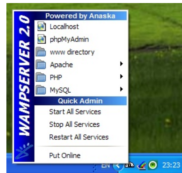
Kontextové menu
