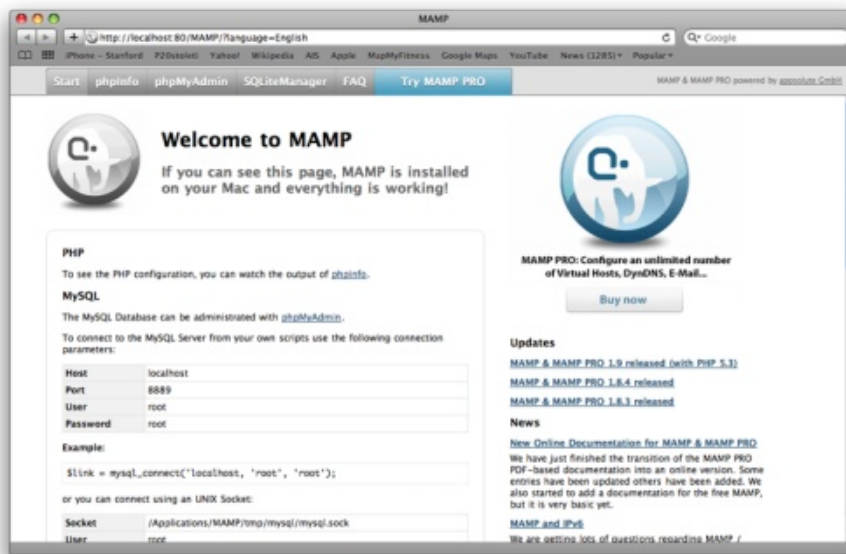
Štartovacia obrazovka
