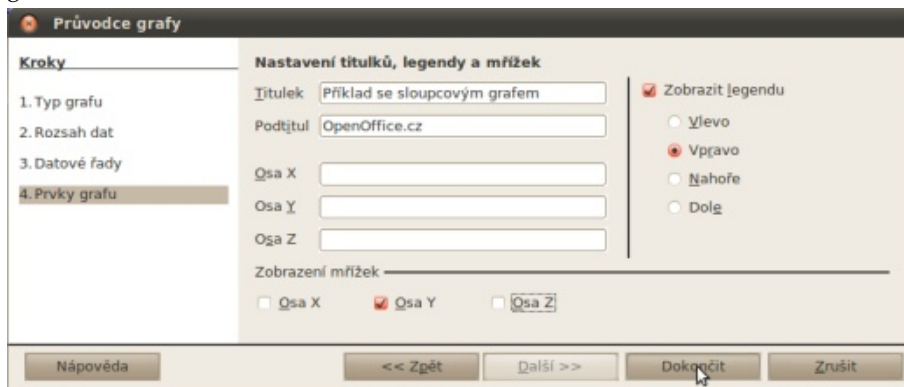
Prvky grafu
