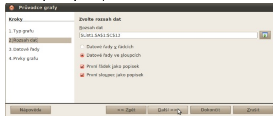
Rozsah dat
