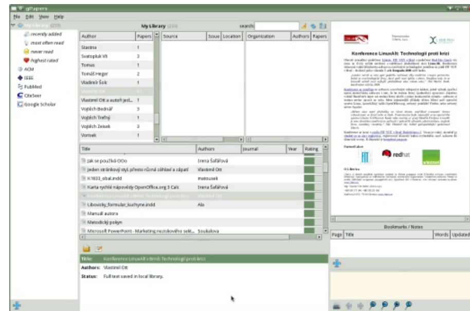
Správa dokumentů
