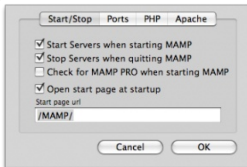
Konfigurácia Start/Stop
